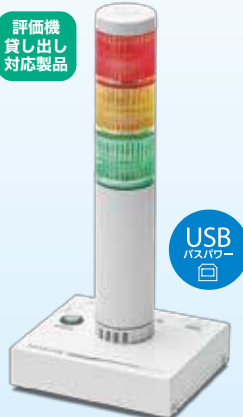
信号灯付インターフェースコンバータ PHE-3FB2-RYG型 RS-232C、USB接続
