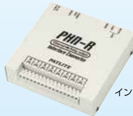
USB バスパワー インターフェース コンバータ PHC-D08型 RS-232C、USB接続 デジタル出力
